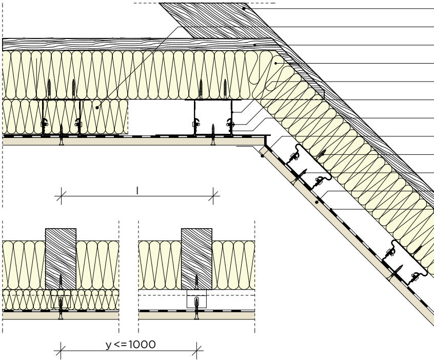
Tetőter vízszintes és ferde síkjának csatlakozása - függesztés direkt függesztővel és állítható kengyellel
