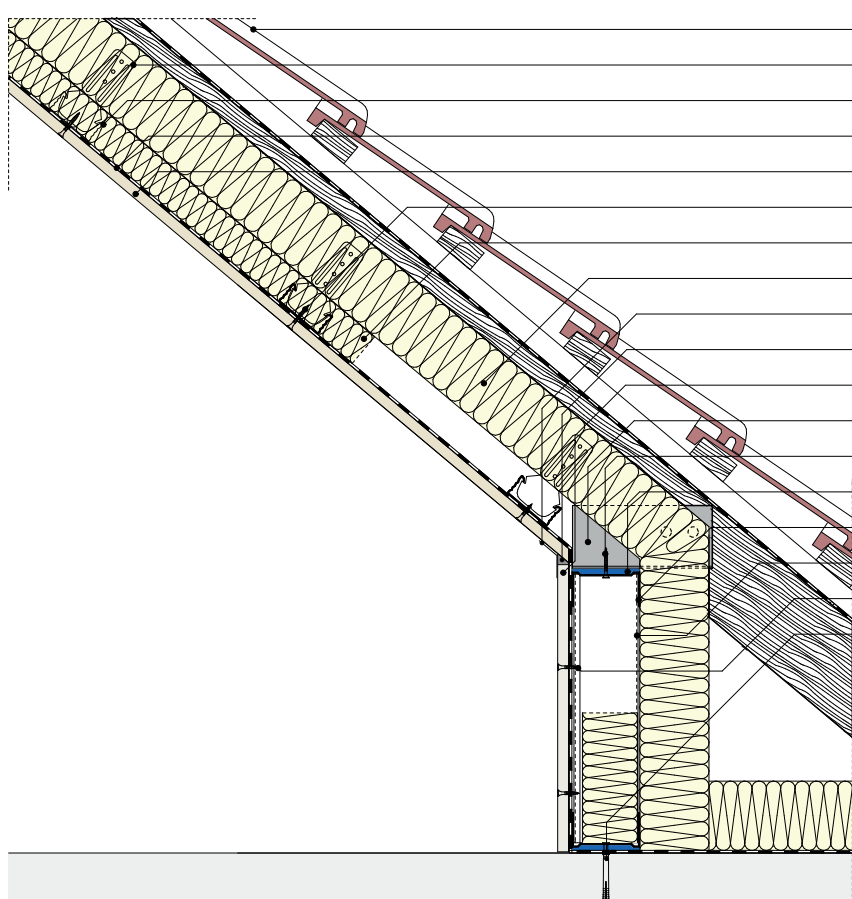
Tetőtér ferde síkjának és szigetelt szerelt térdfalának csatlakozása - függesztés CD-távtartóval
