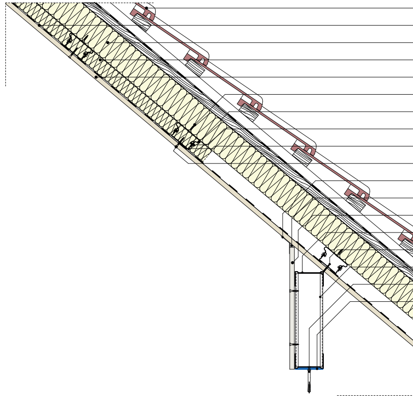
Tetőteri ferde sík és szigetelés nélküli szerelt térdfal csatlakozása - függesztés állítható kengyellel
