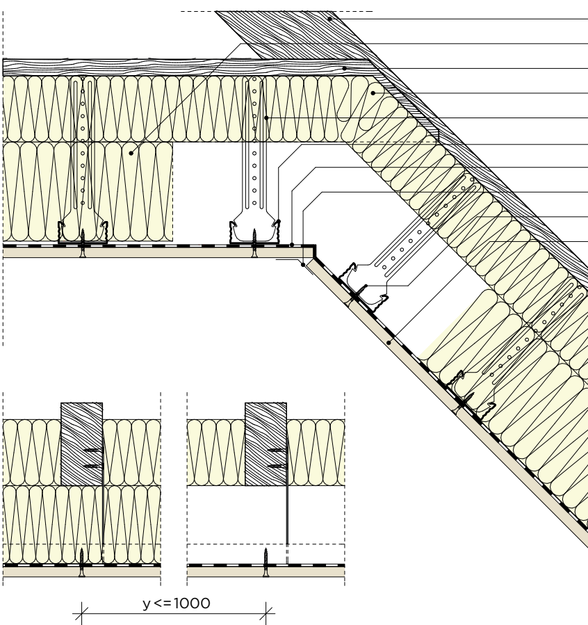
Tetőtér vízszintes és ferde síkjának csatlakozása - függesztés CD-távtartóval
