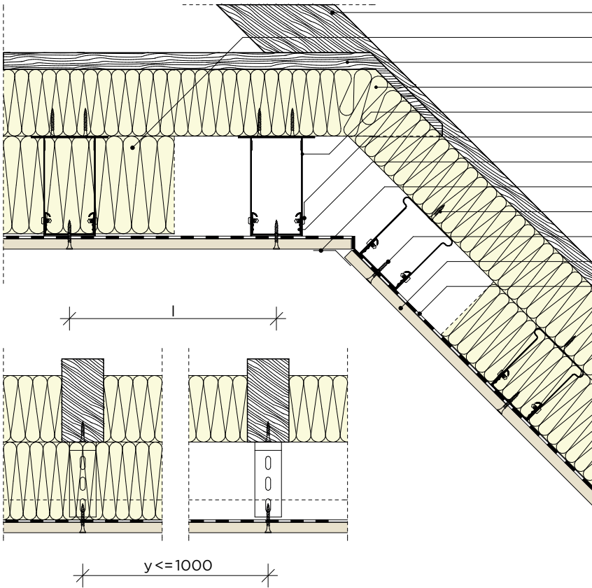
Tetőter vízszintes és ferde síkjának csatlakozása - függesztés direkt függesztővel és állítható kengyellel
