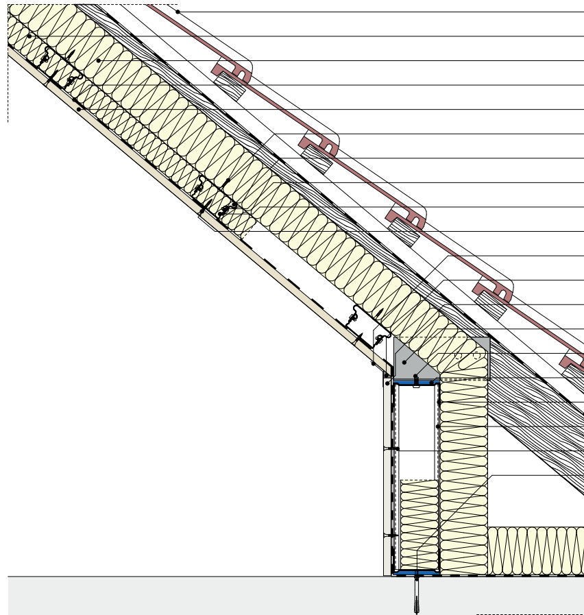
Tetőter ferde síkjának és szigetelt szerelt térdfalának csatlakozása - függesztés állítható kengyellel – tűzgátló tetőter, térdfal kialakítással
