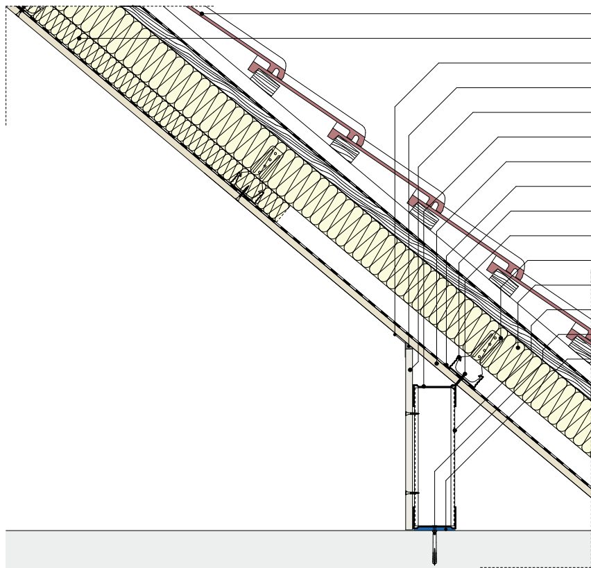
Tetőtér ferde síkjának és szigetelés nélküli szerelt térdfalának csatlakozása - függesztés CD-távtartóval
