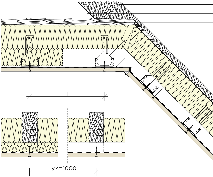
Tetőtér vízszintes és ferde síkjának csatlakozása - függesztés CD-távtartóval
